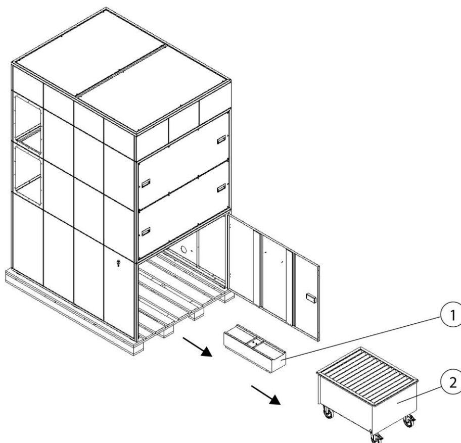
Рис. 16: Извлечение пылесборника и подъемника
