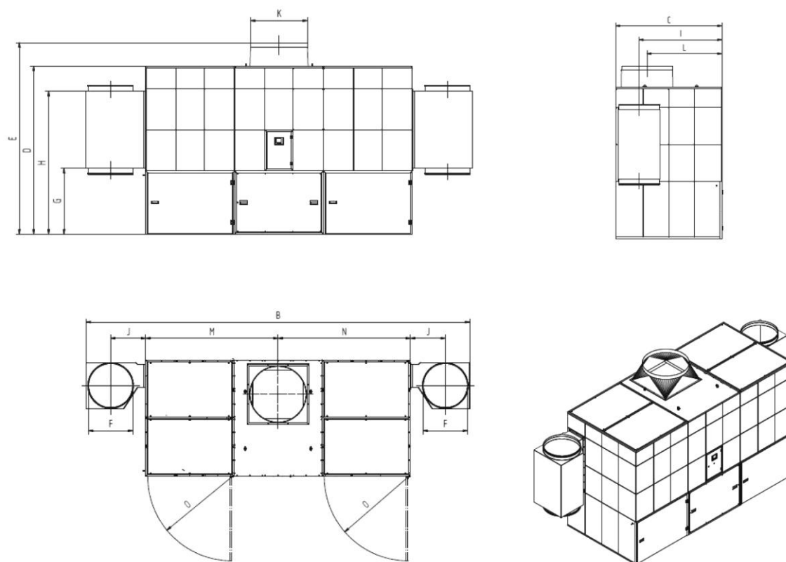
Рис. 79: Габаритный чертеж 34200 + 34220
