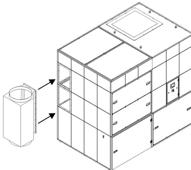
Рис. 26: Монтаж соединительной коробки на стороне всасывания
