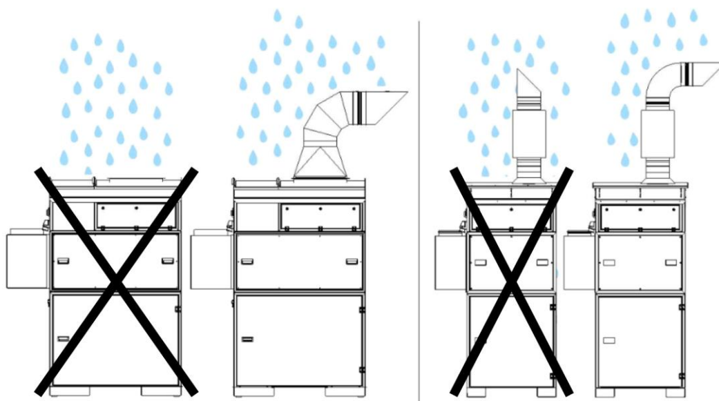
Рис. 5: Версия для наружного применения
