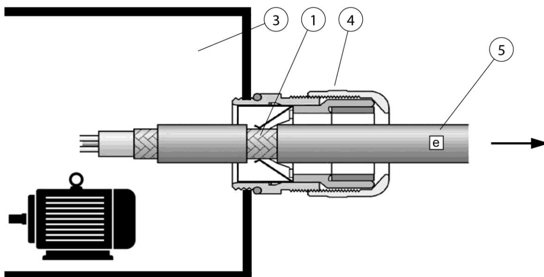
Рис. 37: Присоединение экранирующей плетки кабеля двигателя
