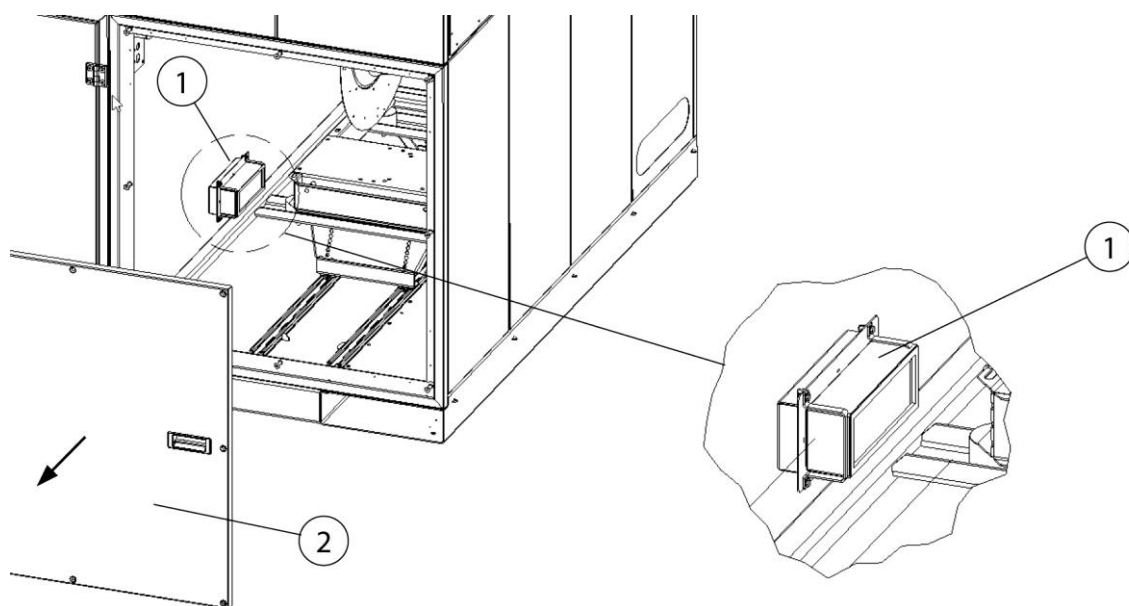
Рис. 58: Доступ к защитному фильтру
