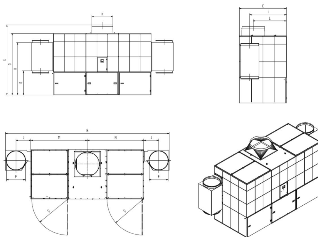
Рис. 77: Габаритный чертеж 34160
