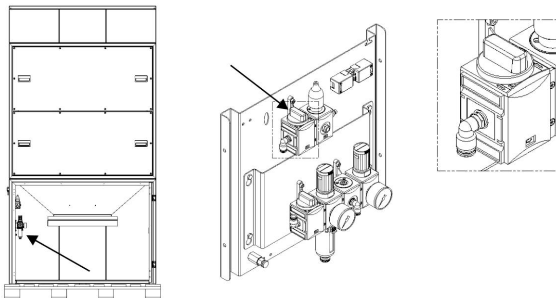
Рис. 14: Клапан опускания пылесборника
