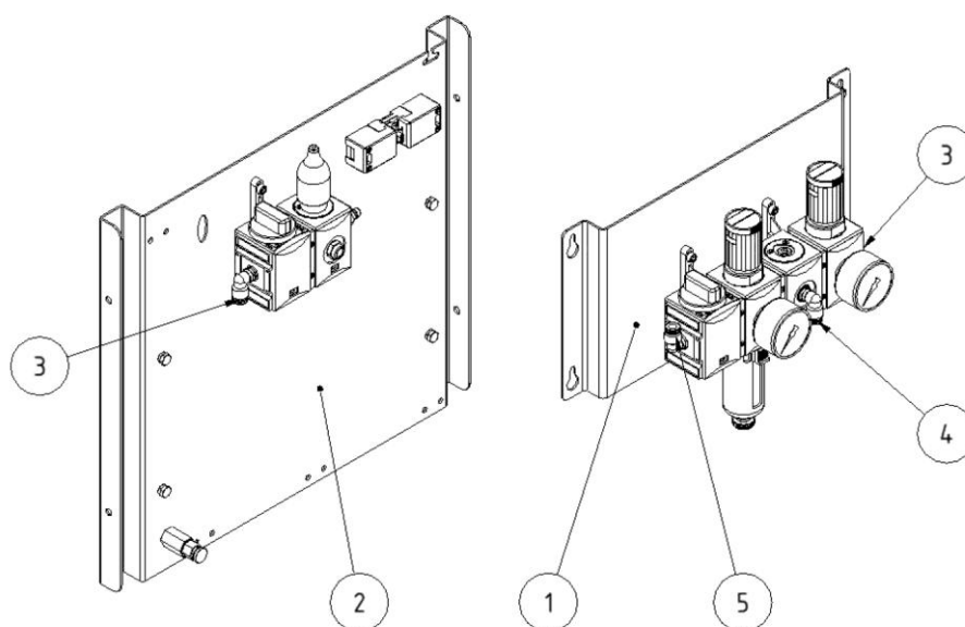
Рис. 31: Узел пневмосистемы
