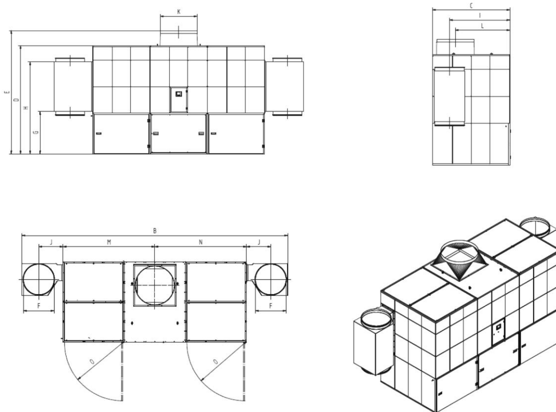
Рис. 78: Габаритный чертеж 34180
