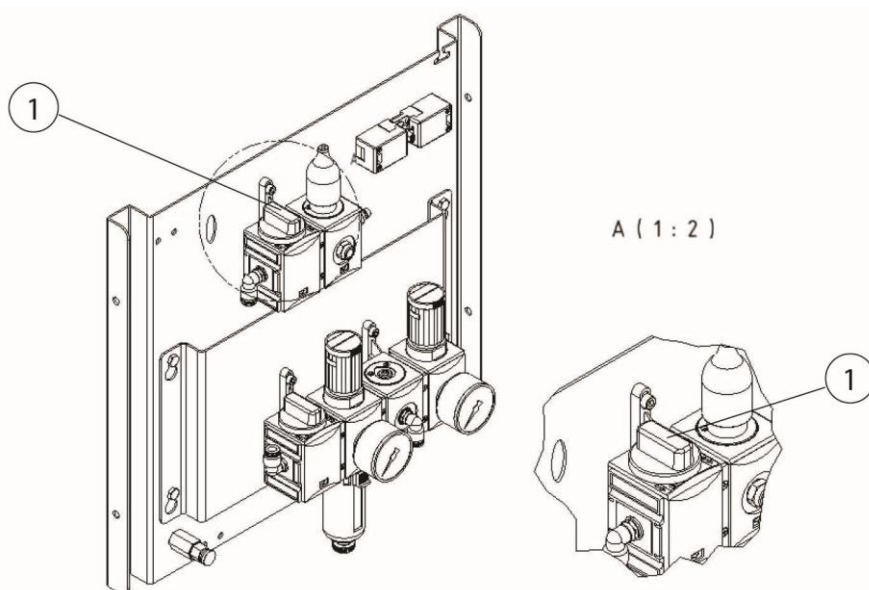
Рис. 55: Пневматический вентиль пылесборника
