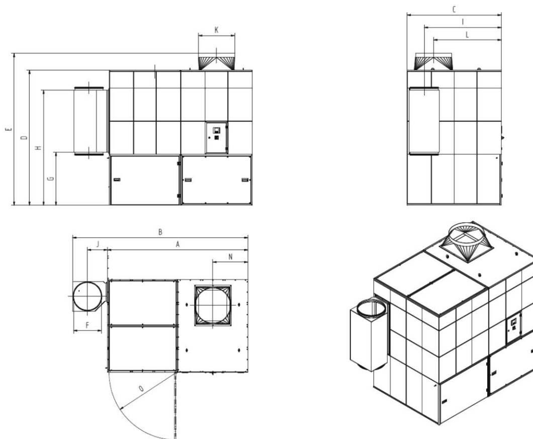
Рис. 76: Габаритный чертеж 34130
