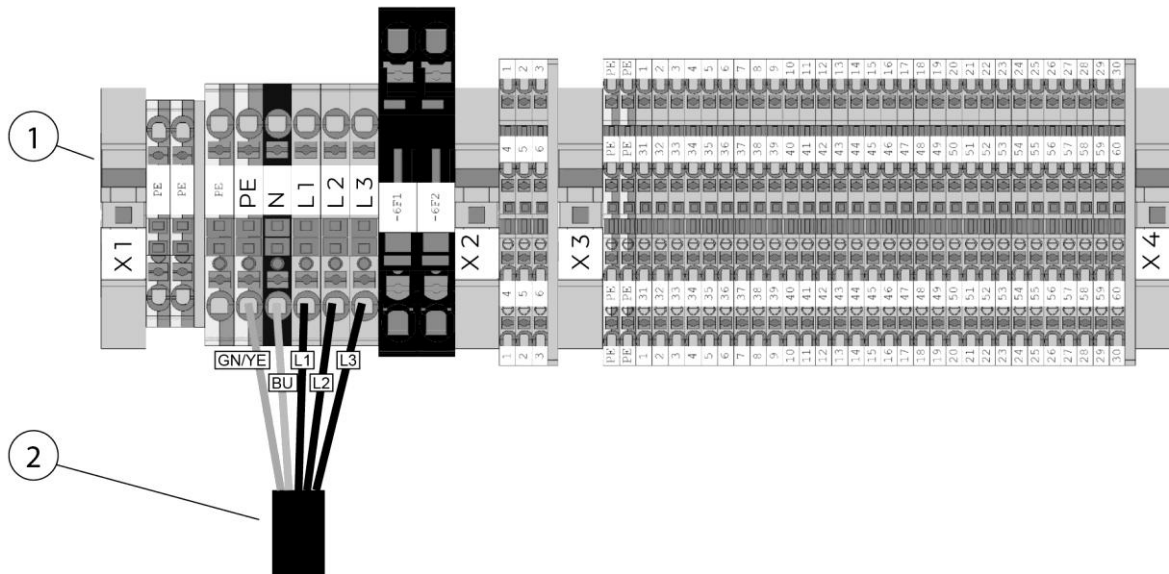
Рис. 32: Рейка с присоединительными зажимами в распределительном шкафу изделия
