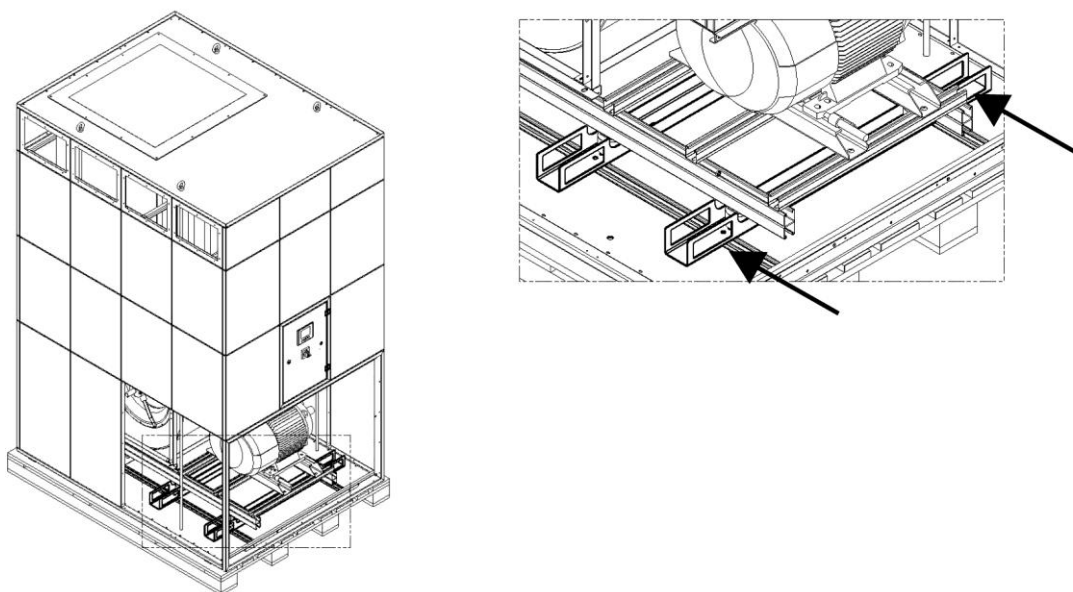
Рис. 11: Подъем вентилятора вилочным погрузчиком
