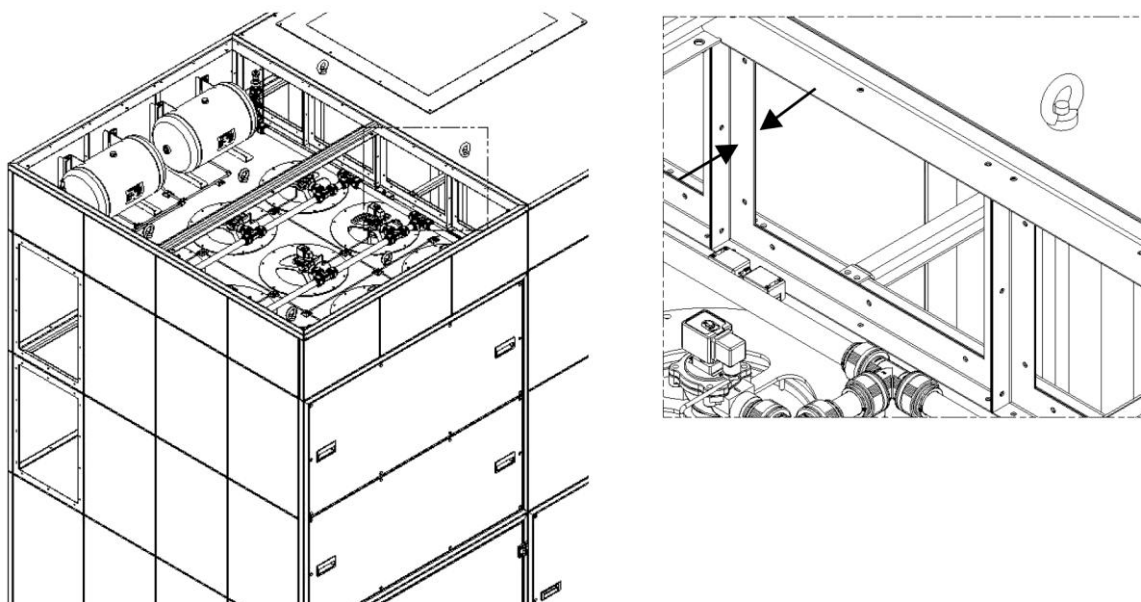
Рис. 21: Соединение вентилятора с фильтром
